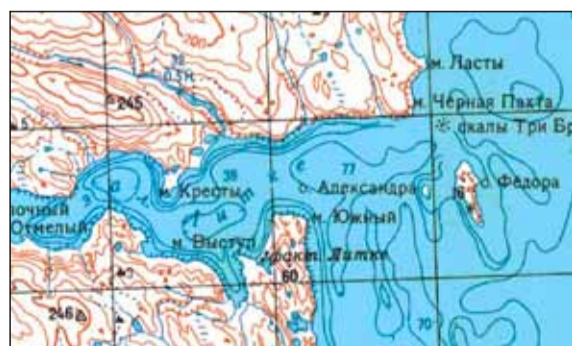
Залив на восточном побережье южного острова Новой Земли и остров Фёдора
